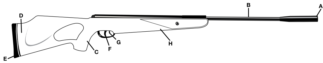
A. Muzzle B. Barrel C. Grip D. Stock E. Butt F. Trigger G. Safety H. Forearm
